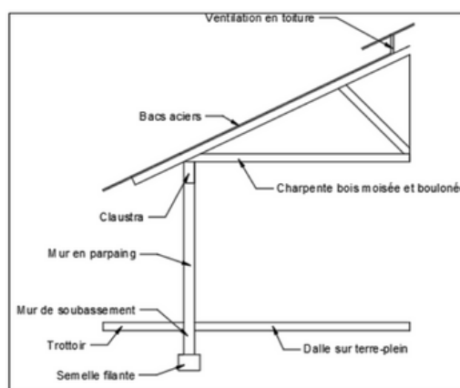
Schéma de principe de construction pour les salles de classe et le réfectoire.
